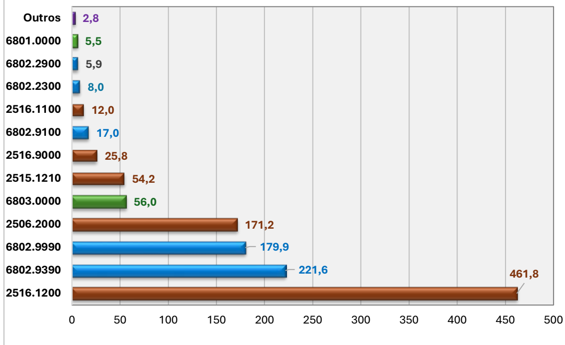
Figura 5 - Exportações brasileiras de rochas naturais, por NCM, de janeiro a julho de 2026 - 1.000 t
