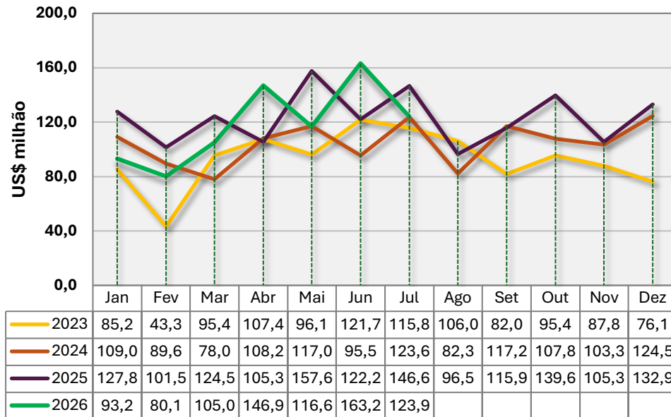
Figura 2 - Exportações brasileiras mensais do setor de rochas ornamentais - 2023-2026
