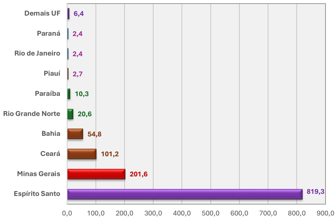
Figura 10 - Principais estados exportadores de rochas naturais de janeiro a julho de 2026 - 1.000 t
